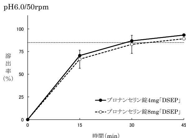
(溶出曲線)
