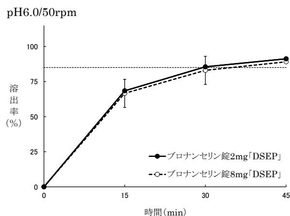
(溶出曲線)
