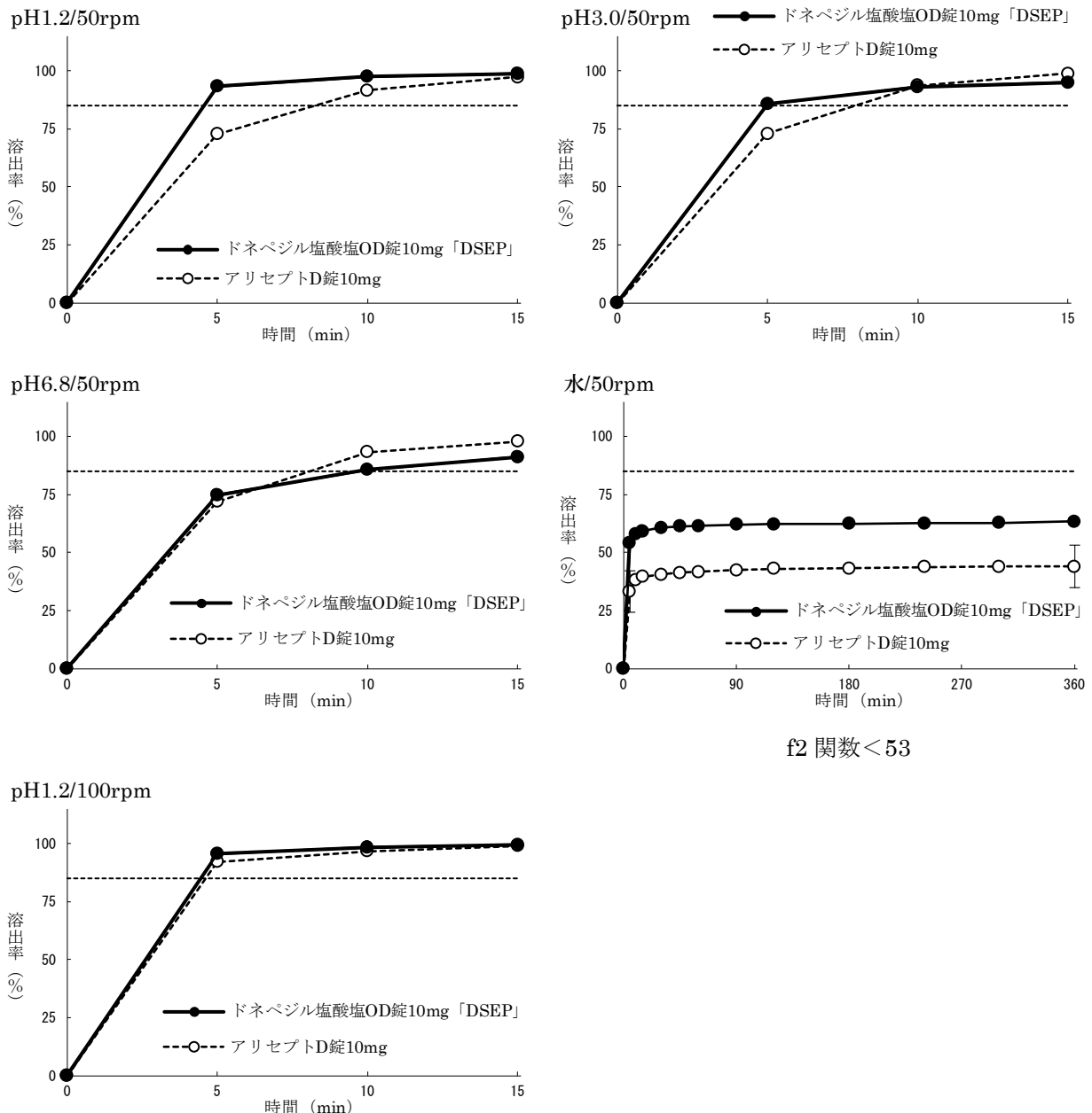
(溶出曲線)
