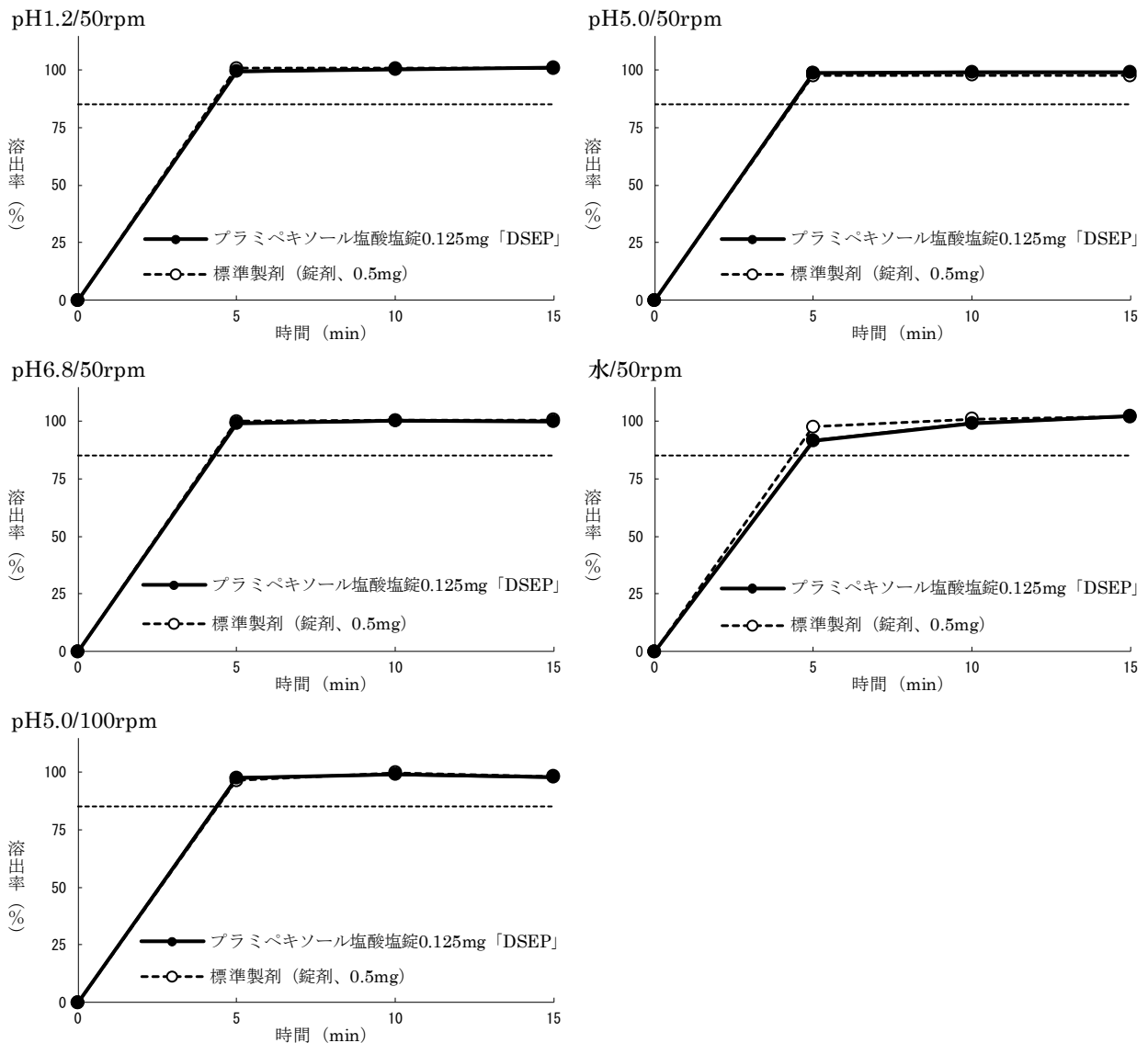
(溶出曲線)
