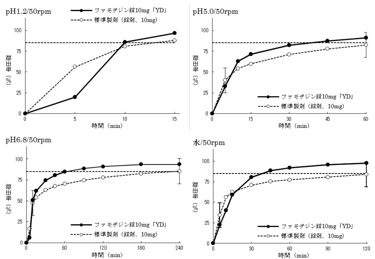
(溶出曲線)
