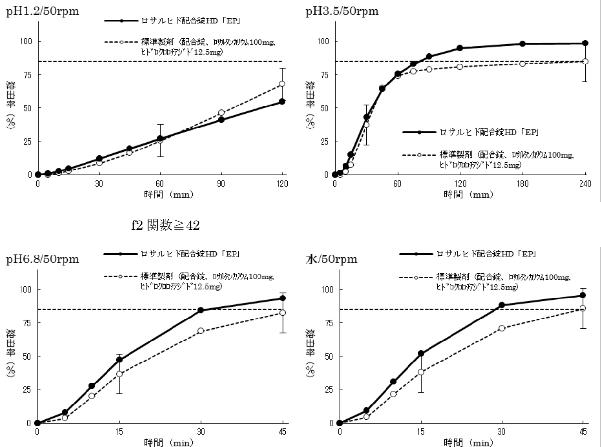
(溶出曲線)
