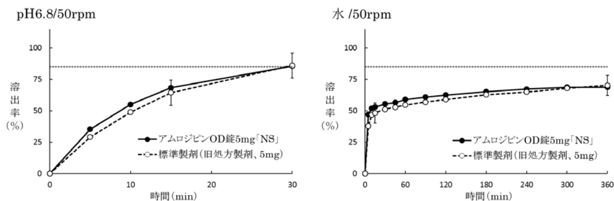
最終比較時点でのアムロジピン OD 錠 5mg 「NS」の個々の溶出率 (%)
