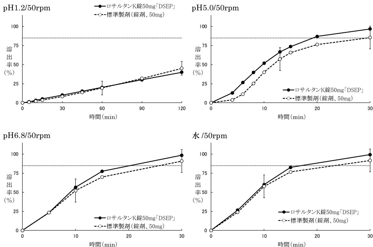
(溶出曲線)
