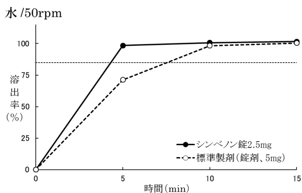
(溶出曲線)
